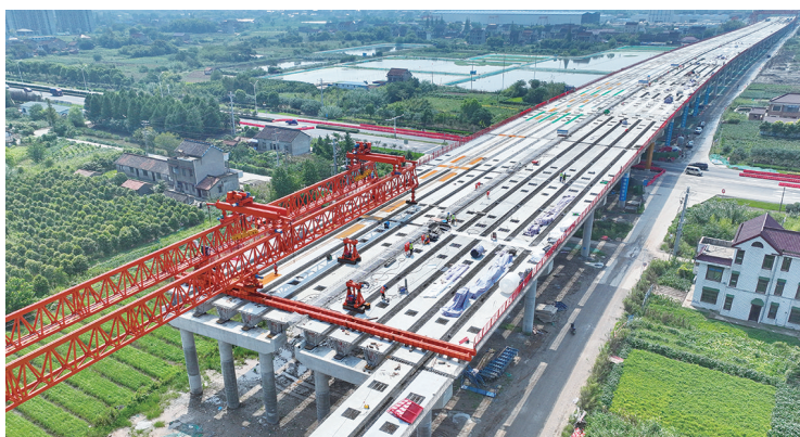
高架桥施工
